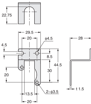
材质: SUS304 M3(长6mm)带垫圈螺丝2个
