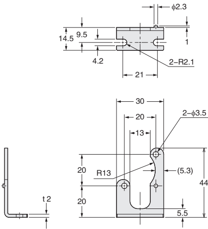
材质: SPCC(光泽镀锌) M3(长6mm)带垫圈螺丝2个
